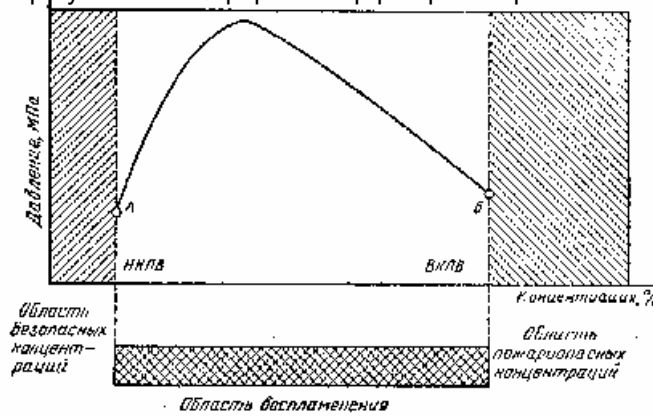
Рис. 5.3 Изменение давления при взрыве газоздушных смесей в зависимости от концентрации горючего вещества
