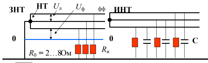
Рис. 3.14 Схемы электрических сетей с ЗНТ и ИНТ
