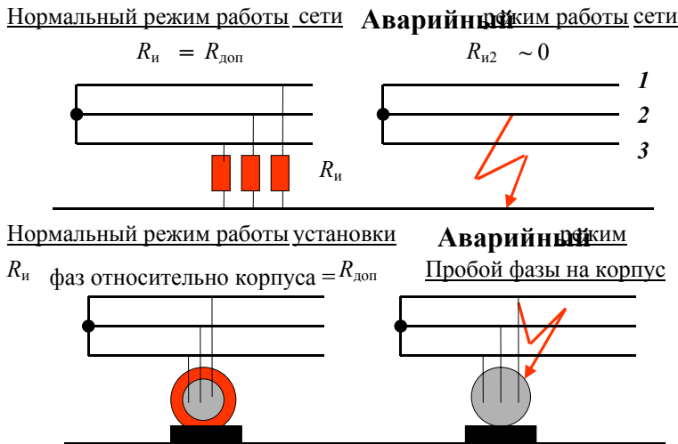
Рис. 3.13 Режимы работы сети и электроустановки
